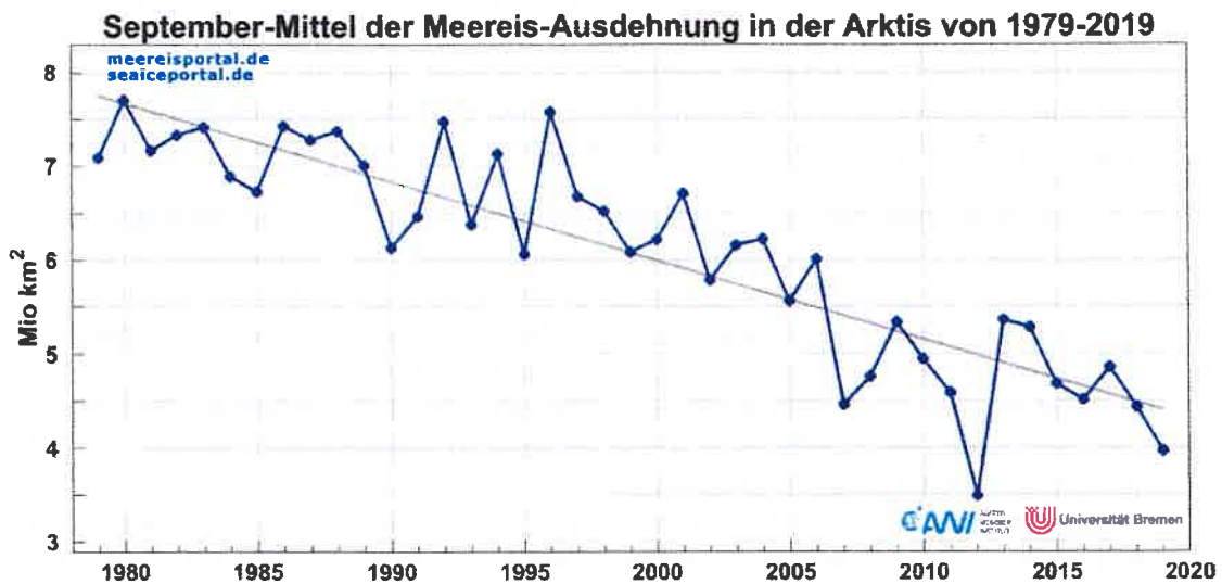
Abb. 5: Rückgang der sommerlichen Meereisausdehnung in der Arktis.
