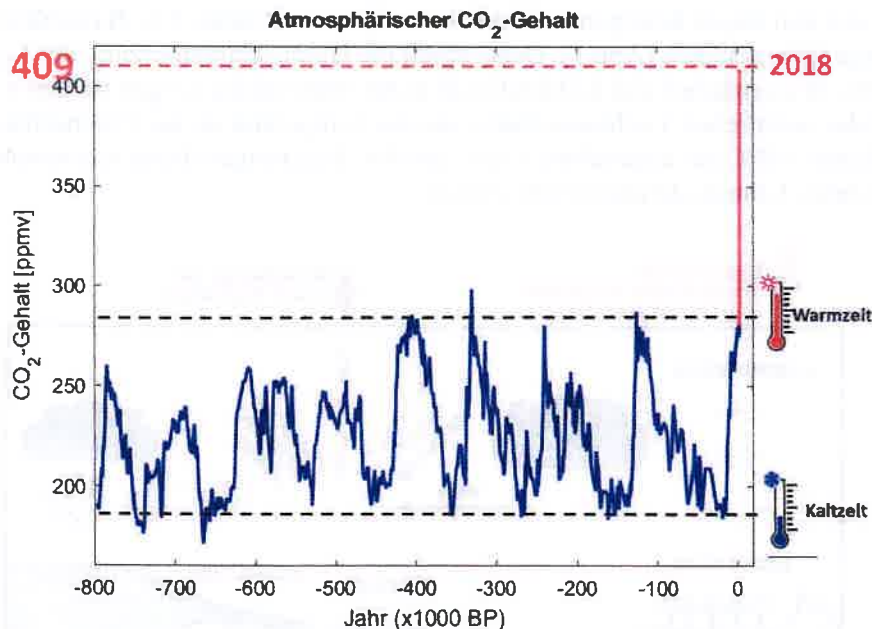
Abb. 2: CO 2 -Gehalt der Luft seit 800.000 Jahren, ermittelt aus Lufteinschlüssen im EPICA Dome C (Antarktische) Eiskern (blau, Lüthi, D. et al., 2008) und direkten Messungen von Luftproben (seit 1958, rot, Datenquelle: www.esrl.noaa.gov/gmd/ccgg/trends/ ).
